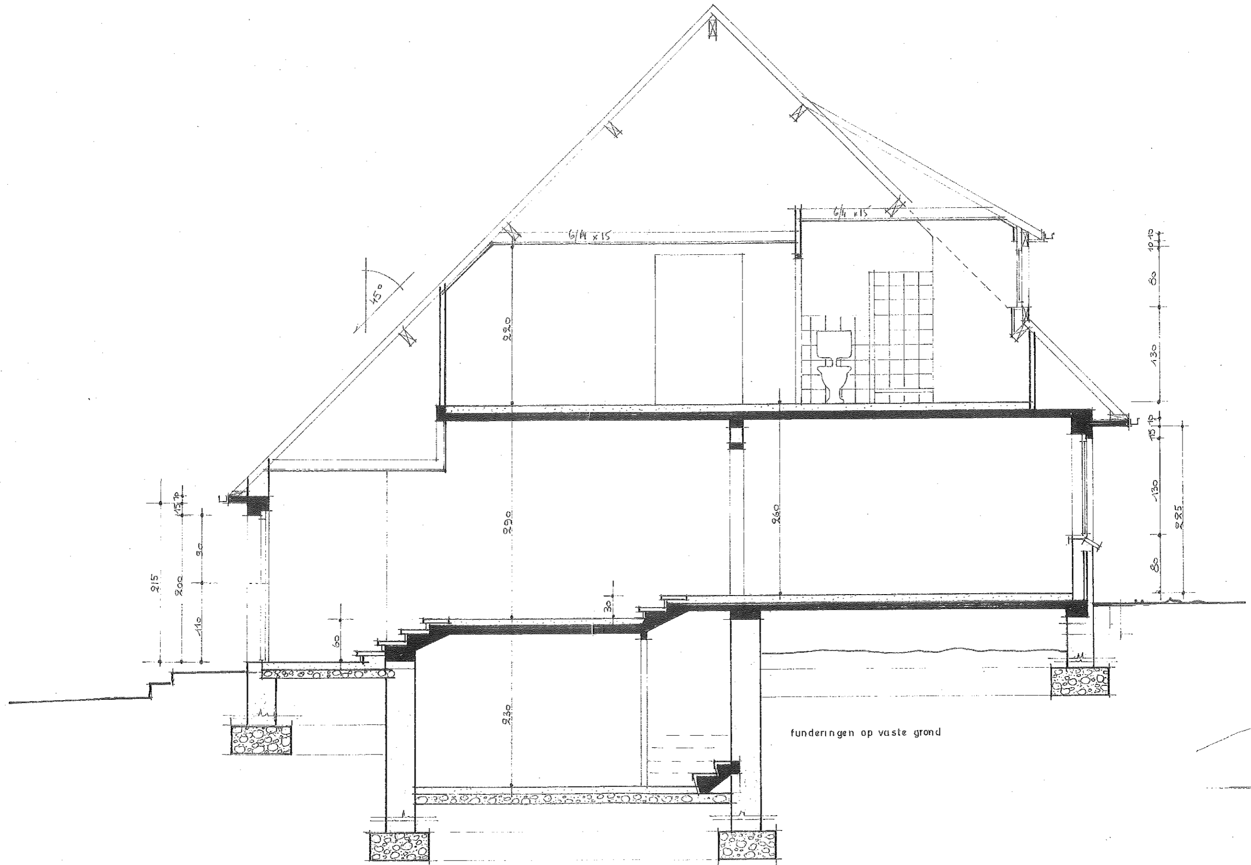
DOORSNEDE A A'
